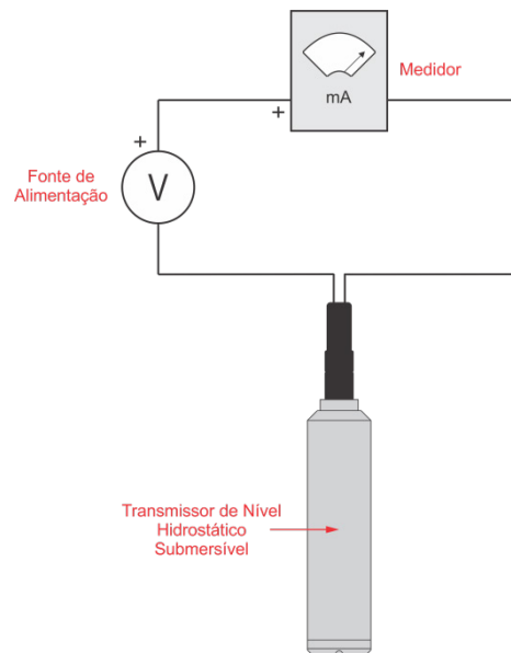
Fig. 05 – Conexões elétricas
