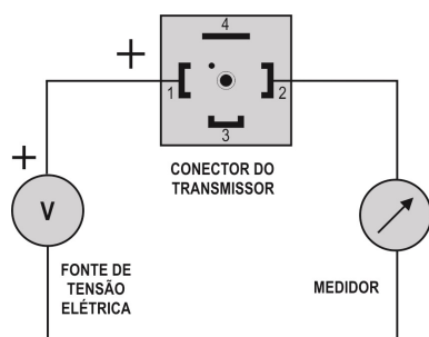
Figura 2 – Conexões elétricas
