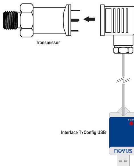
Figura 3 – Conexão do TxConfig-USB
