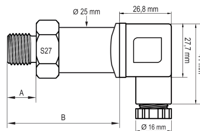
Figura 5 – Dimensões do transmissor (**)
