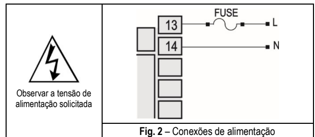
Fig. 2 – Conexões de alimentação
