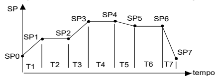
Fig. 9 - Exemplo de programa de rampas e patamares
