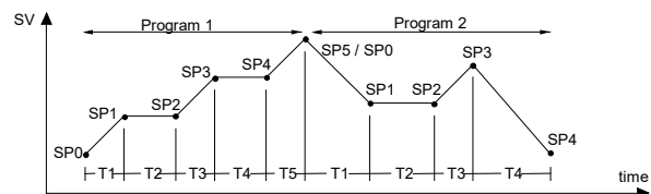
Fig. 11 - Exemplo de programa 1 e 2 interligados
