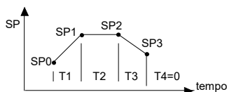
Fig. 10 - Exemplo de programa com poucos segmentos
