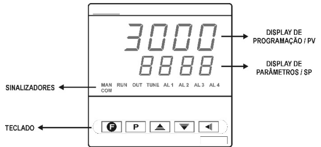
Fig. 8 - Identificação das partes do painel frontal
