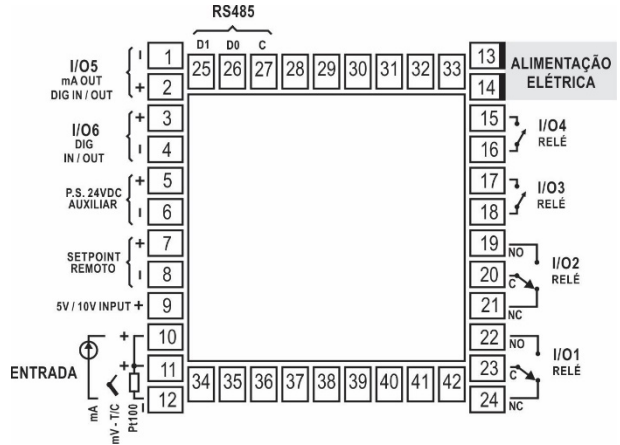
Fig. 1 - Conexões do painel traseiro.
