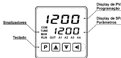
Figura 7 - Identificação das partes do painel frontal
