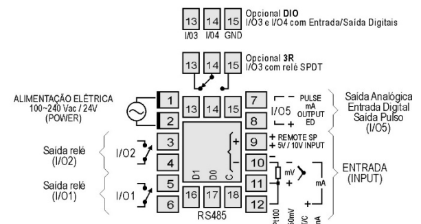
Figura 1 - Conexões do painel traseiro
