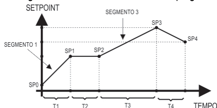
Fig. 03 - Exemplo de programa de rampas e patamares
