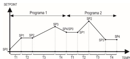
Fig. 04 - Exemplo de programas interligados
