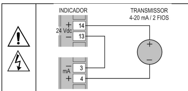
Figura 05 – Exemplo de utilização da fonte de tensão auxiliar do indicador
