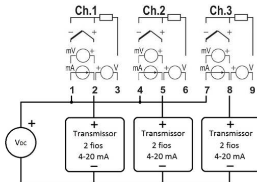
Figura 21 Fonte auxiliar para alimentação de transmissores 4-20 mA (2 fios)
